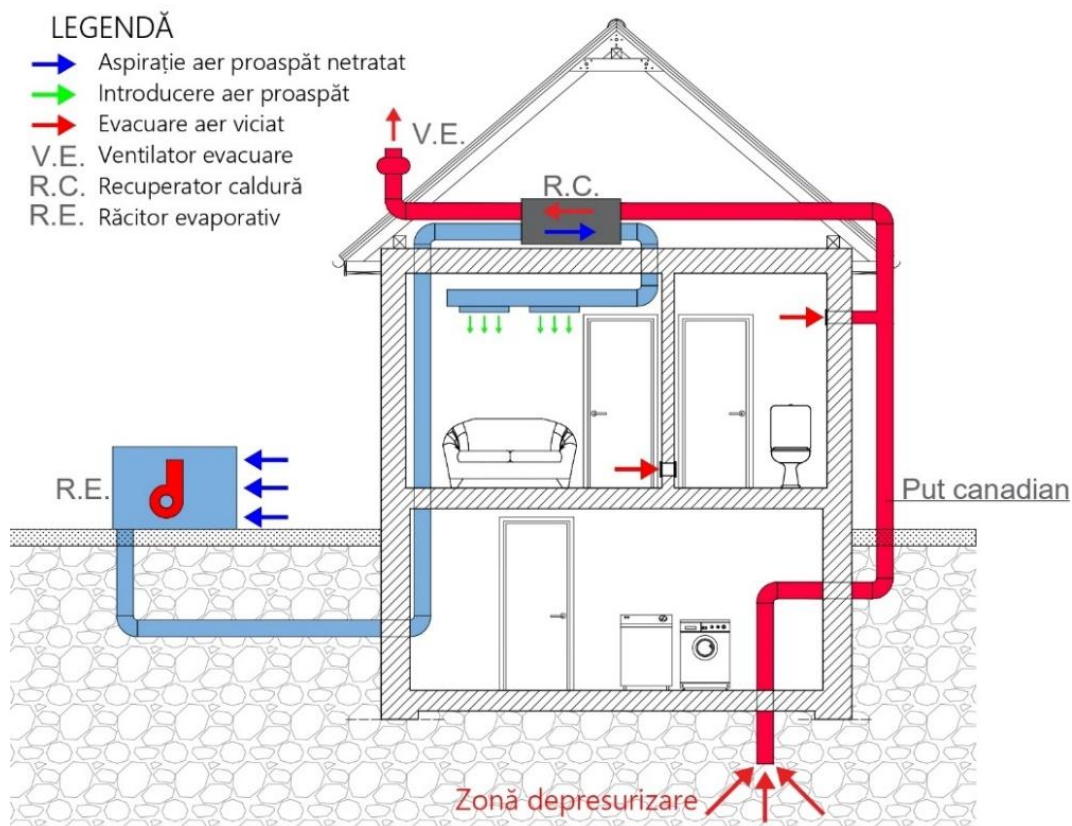
Figura 36 - Sistem de ventilare mecanică centralizată cu recuperare de căldură, depresiune sol și răcitor evaporativ - Schema de principiu
