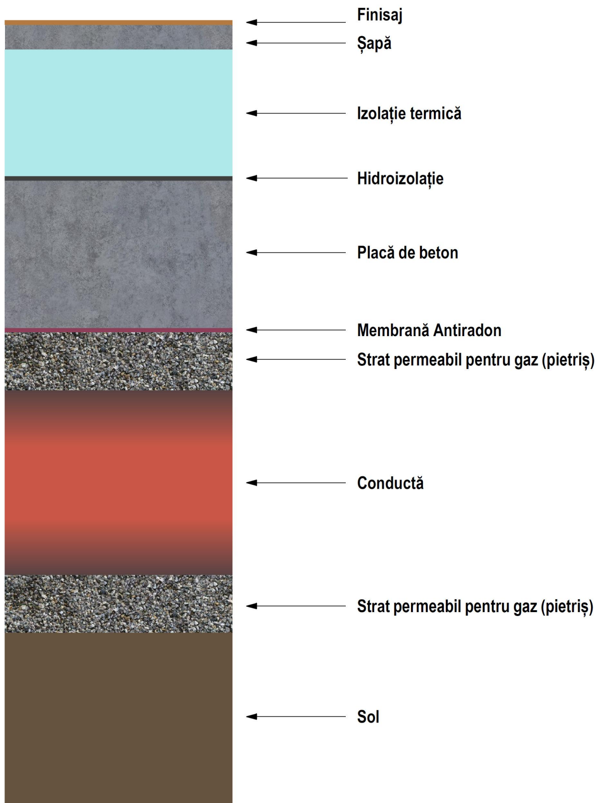
Figura 52 Recomandare privind stratificația pentru izolarea plăcii pe sol.
