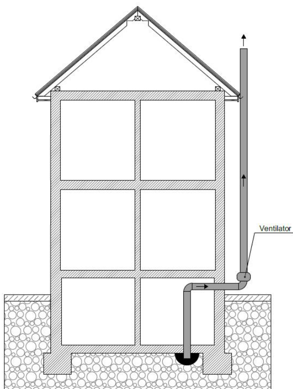
Figura 13 - Depresurizarea solului sub placă cu ventilator exterior clădirii și evacuare la nivelul acoperișului de la subsol- Schema de principiu
