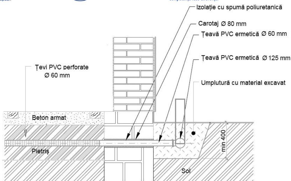
Figura 7 - Secțiune plan de instalare a unei metode de depresurizare activă a solului (DAS) - Schema de principiu
