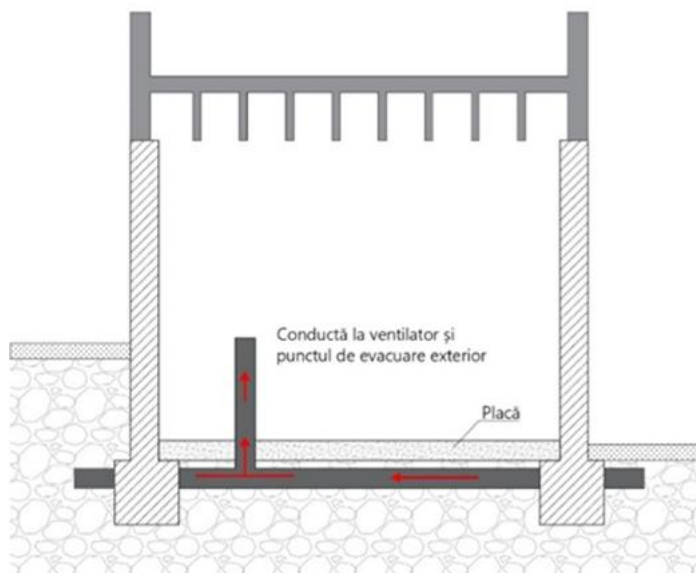
Figura 9b) Depresurizarea solului sub tubulatura de drenaj - Schema de principiu
