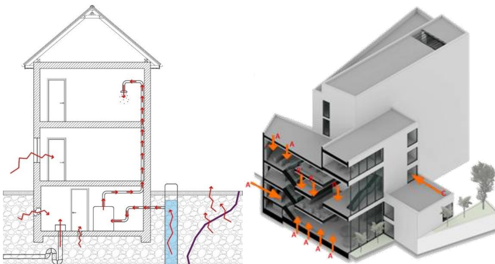
Figura 1 - Surse și căi de intrare a radonului în clădiri - Schema de principiu
