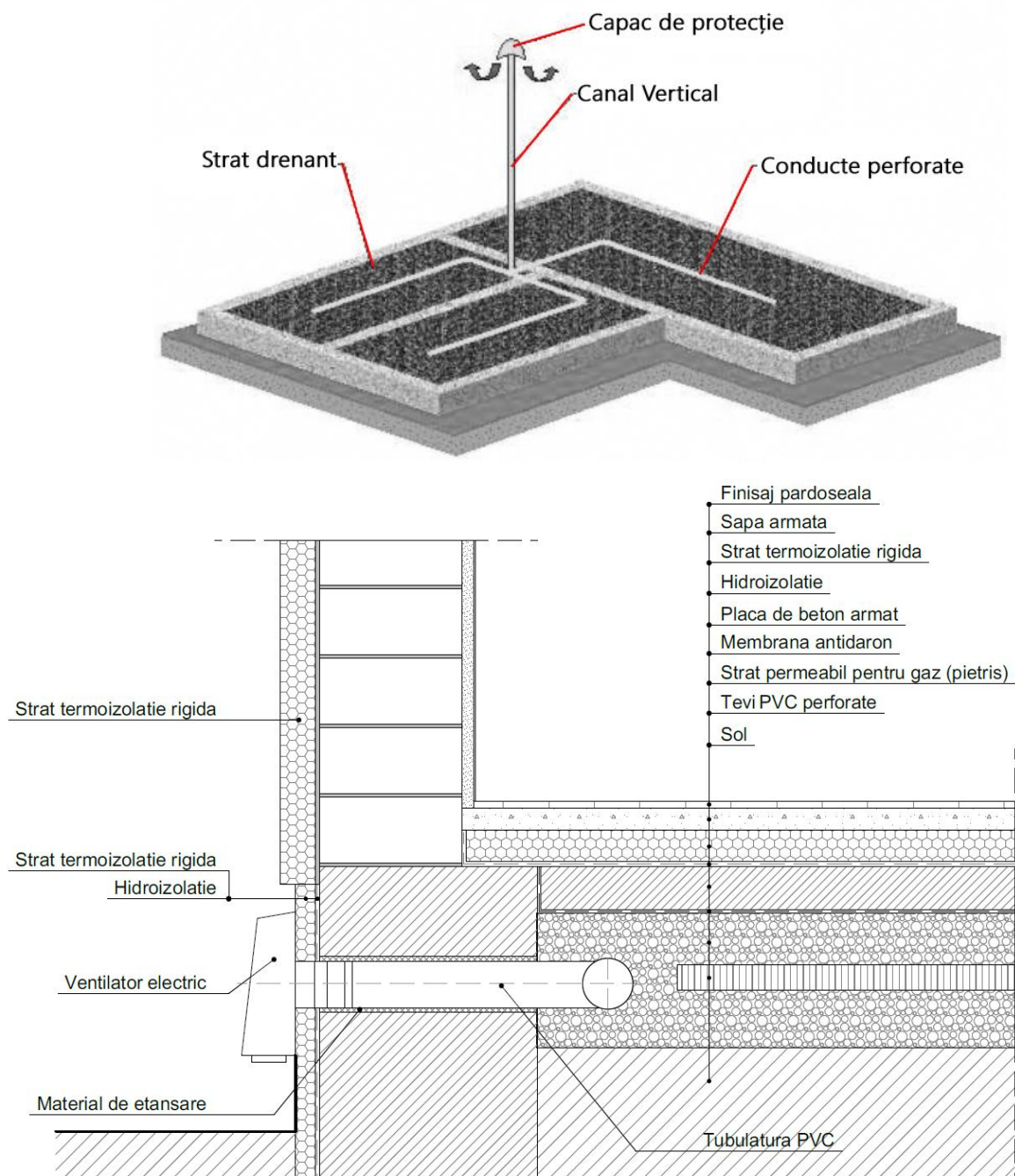
Figura 41 - Reducerea presiunii prin sisteme de conducte perforate
