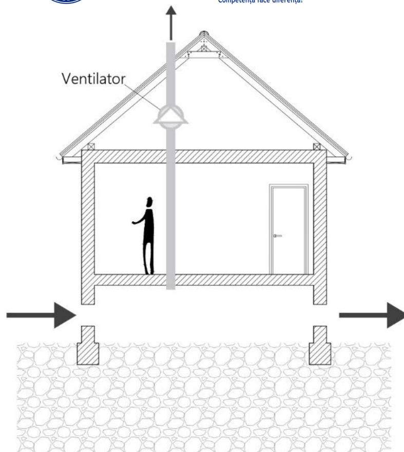
Figura 47 - Schema de principiu - Ventilarea mecanică a spațiului tehnic închis cu sistem vertical de conducte de aer și ventilator de aspirație
