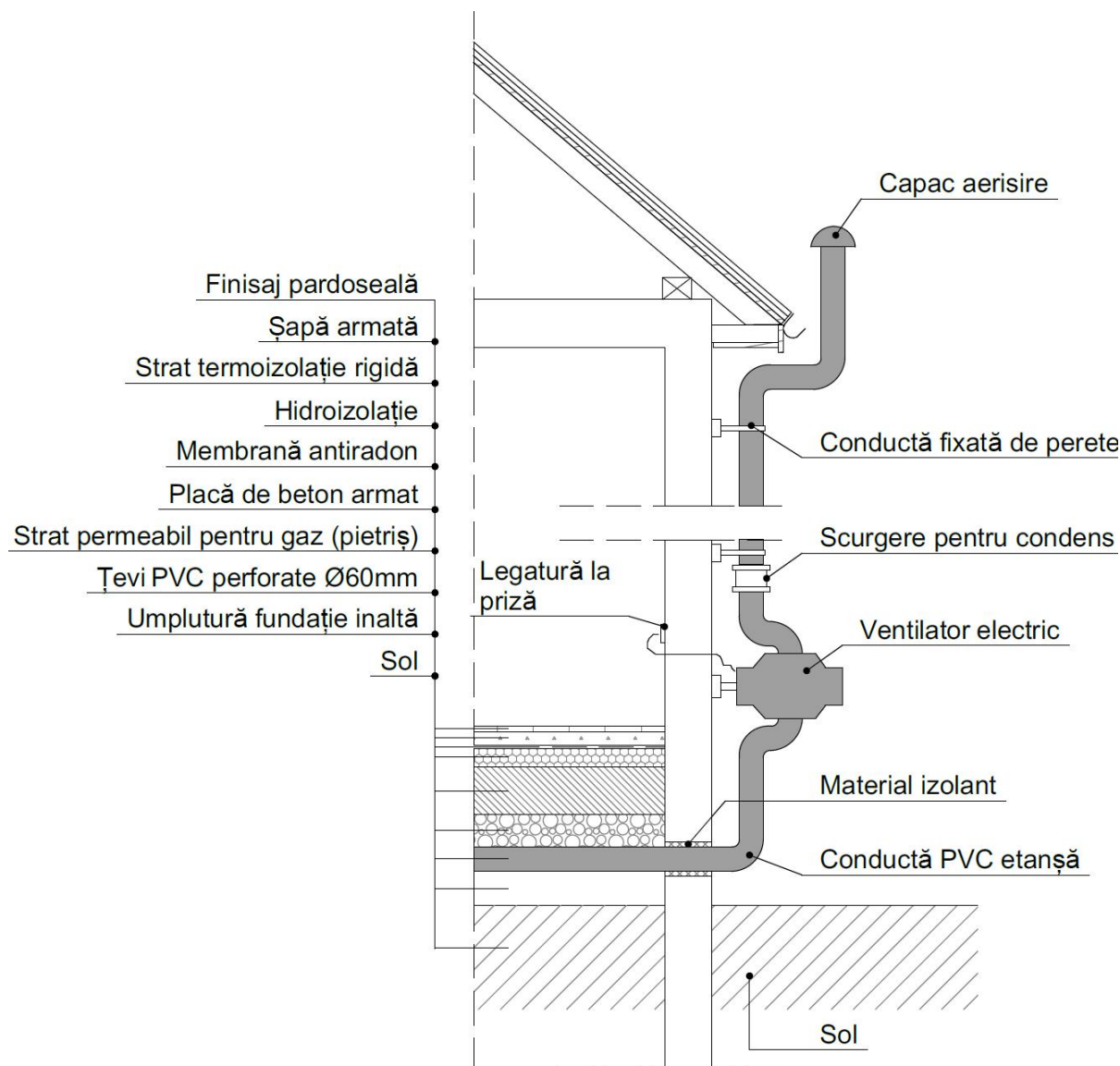
Figura 22 - Secțiune de principiu - metodă combinată de remediere a concentrației de radonului - Depresurizarea activă a solului cu izolarea și etanșeizarea fundației și a planșeului, cu aplicarea membranei împotriva radonului la partea superioară a plăcii de beton
