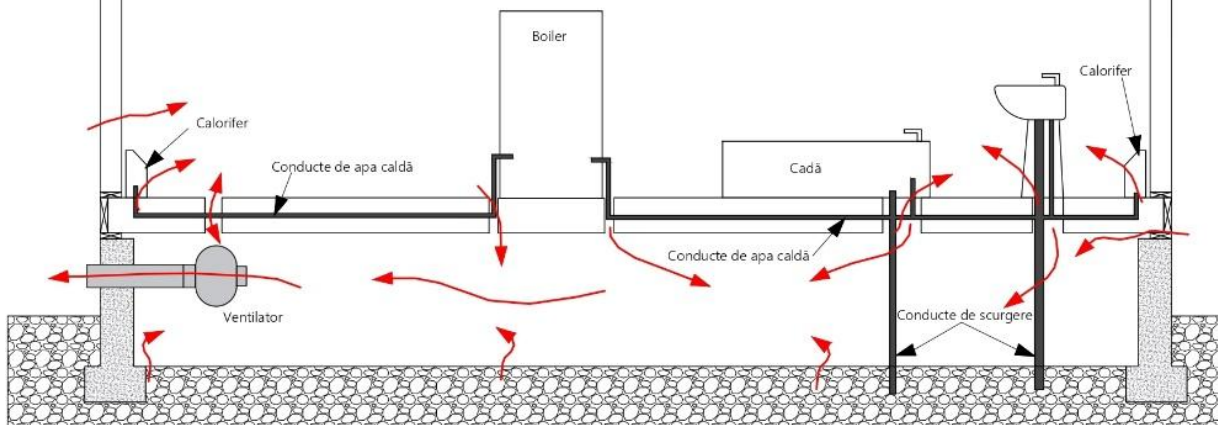
Figura 25 - Schemă de principiu și montaj sistem de ventilare cu presurizare/depresurizare subsol
