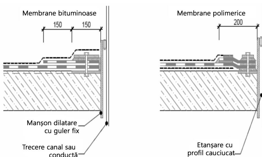
Figura 50 - Etanșarea rosturilor de dilatare - Schema de principiu
