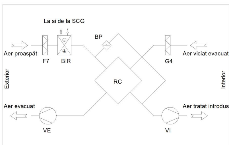
Figura 34 - Schemă de principiu sistem de ventilare cu recuperare de căldură combinat cu sistem de geotermal (colector orizontal) și depresurizare sol
