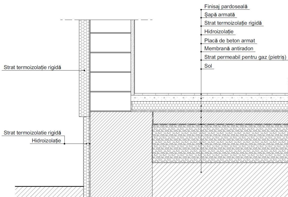
Figura 39 - Aplicarea membranei antiradon/ barierei antiradon la nivelul rosturilor și al contactului perete - pardoseală - Schemă de principiu
