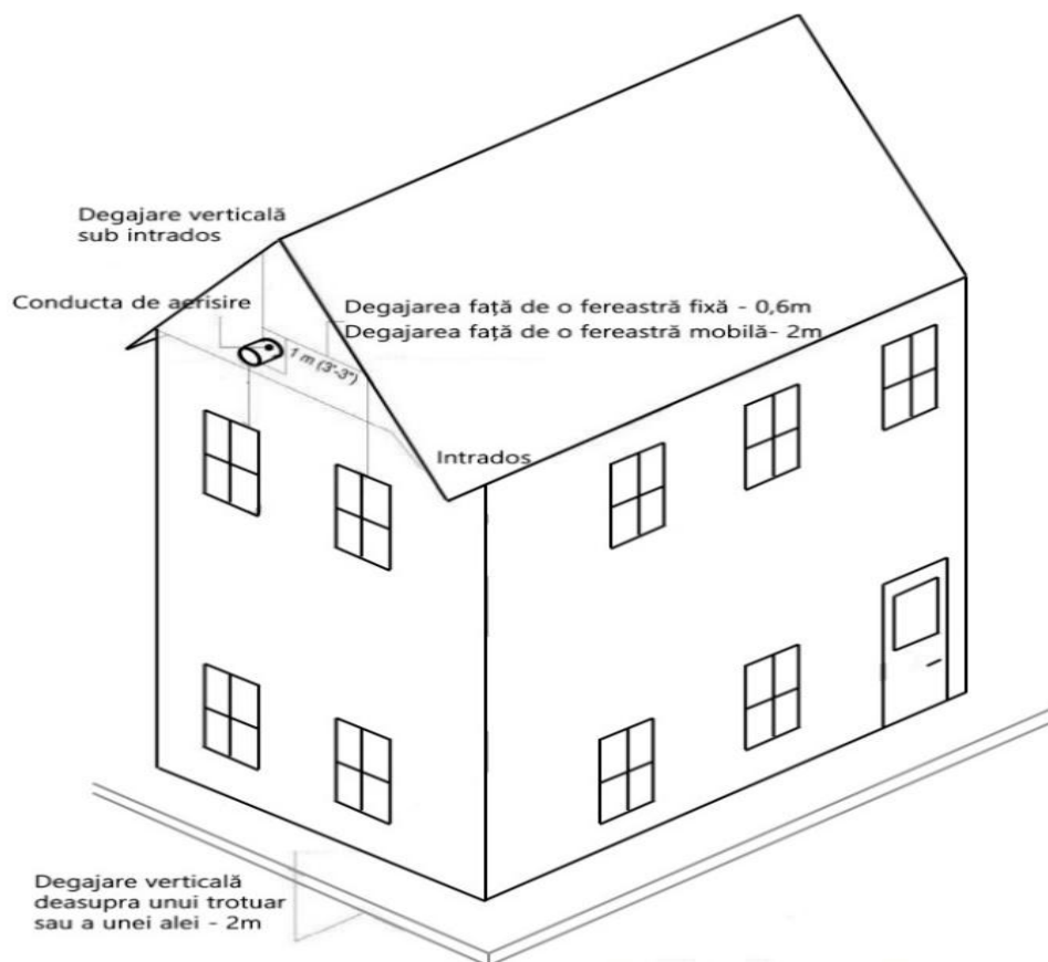
Figura 18 - Sistem de depresiurizare activă cu descărcare la nivelul frontonului - Schema de principiu
