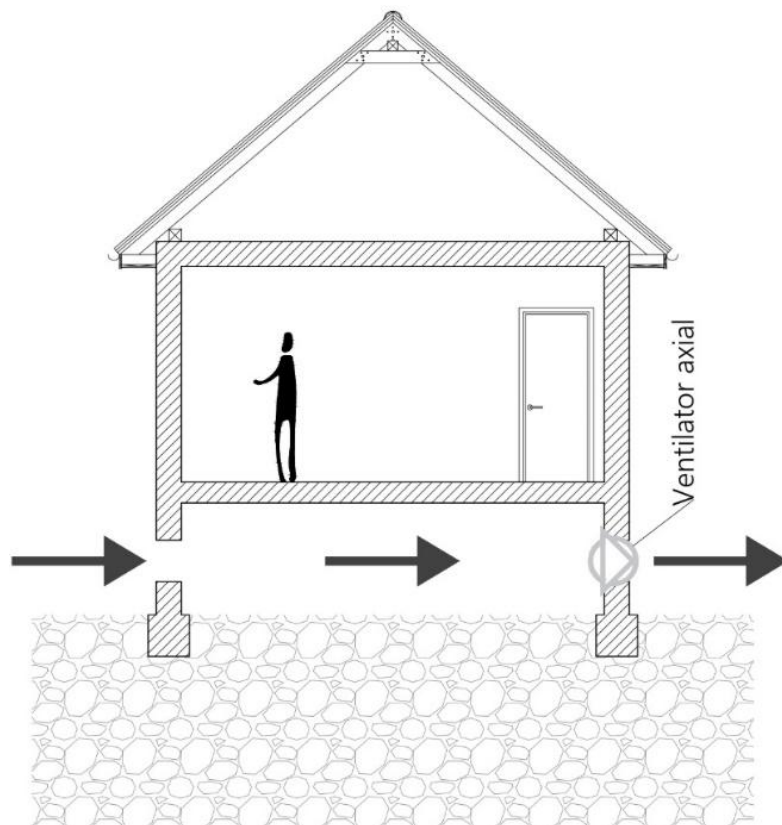
Figura 46 - Schema de principiu - Ventilarea mecanică a spațiului tehnic închis cu un sistem de ventilație prin aspirație amplasat pe un perete
