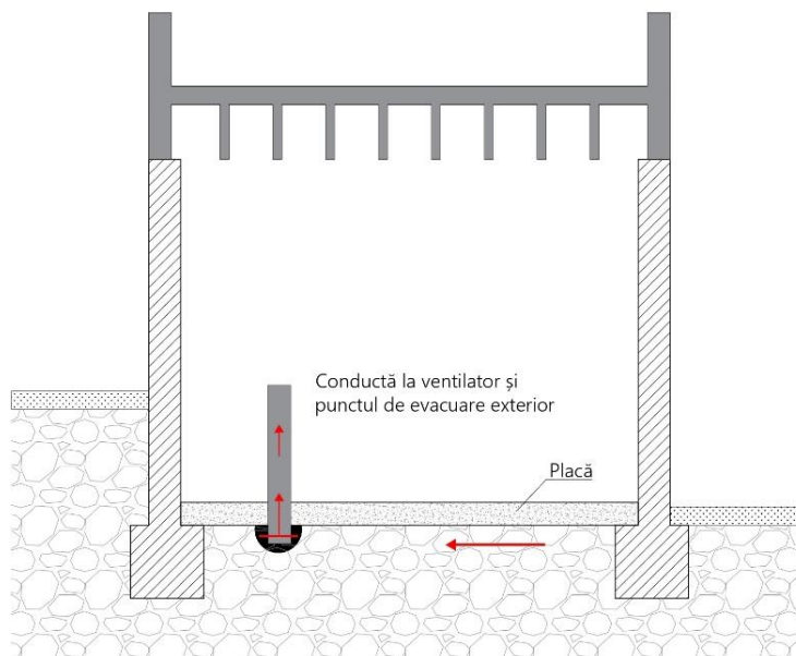
Figura 8- Depresurizarea solului sub placă - Schema de principiu
