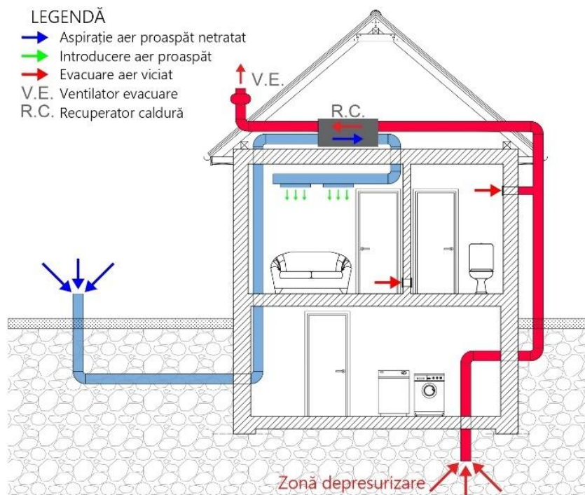
Figura 33 - Imagine reprezentativă cu sistem de ventilație cu recuperare de căldură combinat cu puț canadian și depresurizare sol - Schema de principiu
