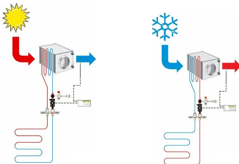
Figura 35 - Sistem de ventilare cu recuperare de căldură combinat cu sistem de geotermal (colector orizontal) și depresurizare sol - Schema de principiu
