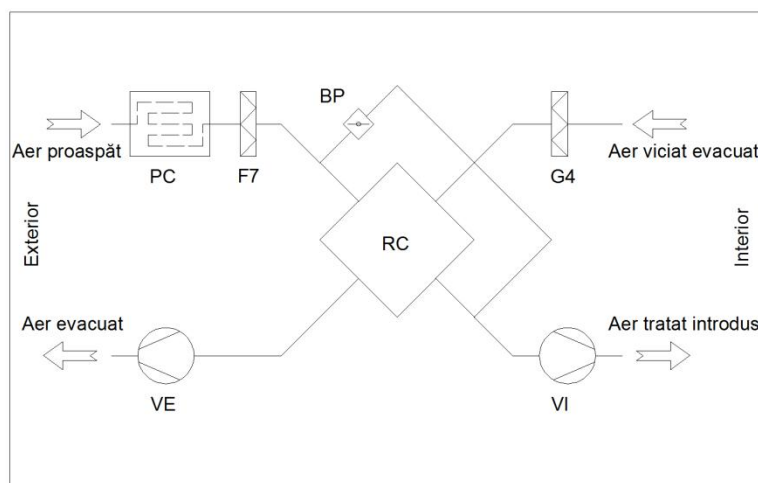
Figura 32 - Schemă de principiu sistem de ventilare cu recuperare de căldură combinat cu puț canadian și depresurizare sol
