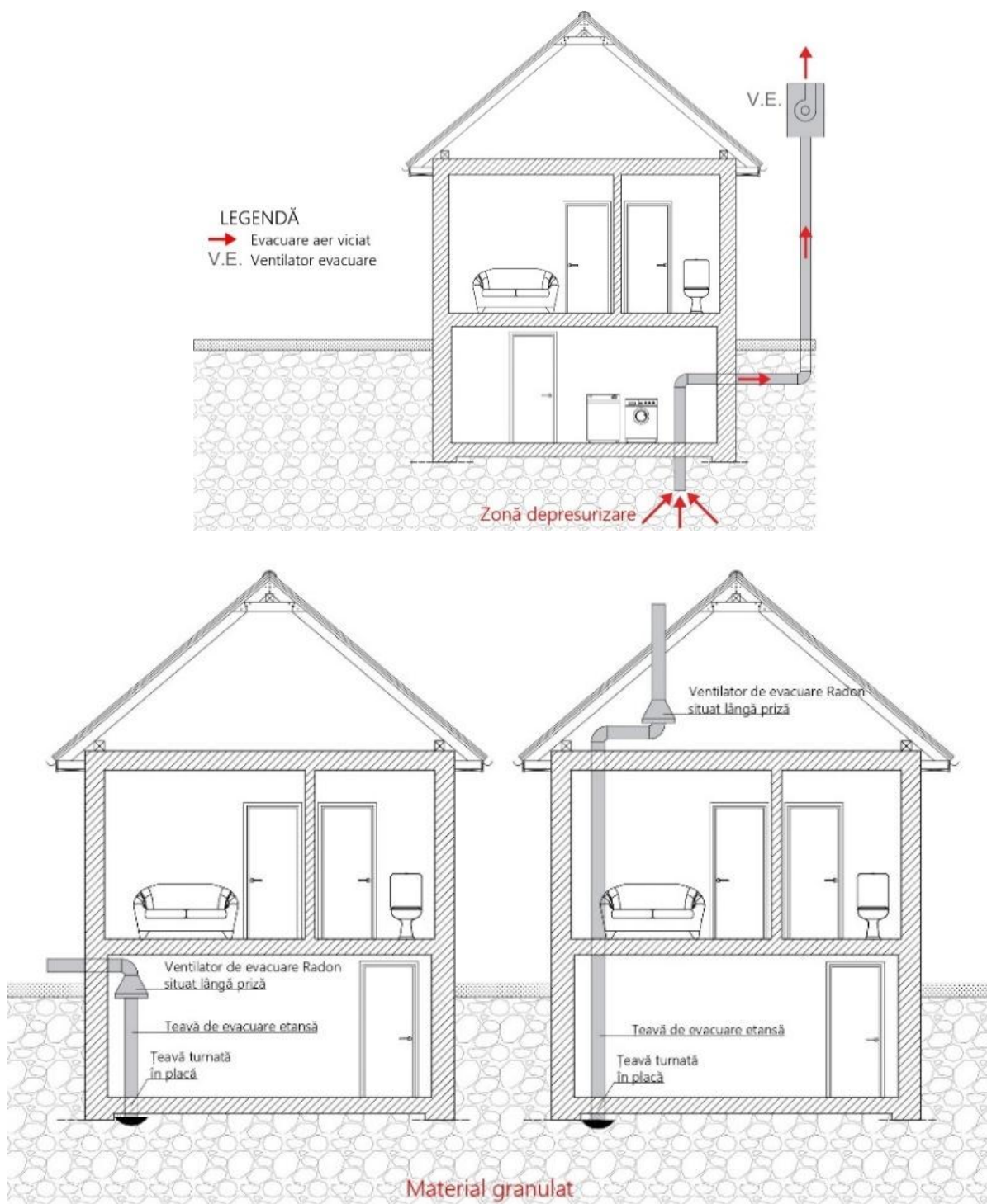
Figura 24 - Sistem depresurizare activă a pardoselii - Schema de principiu
