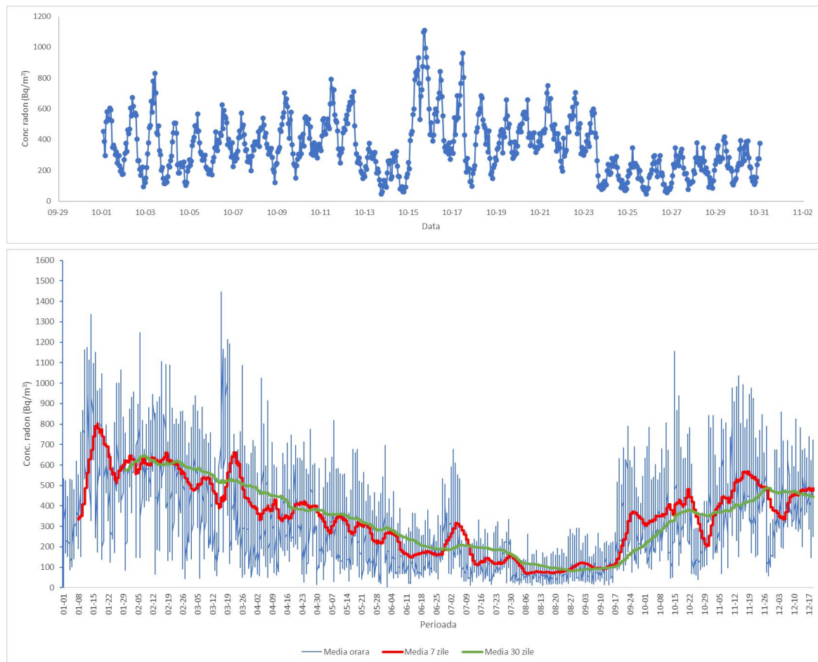
Figura 3 - Exemplu de variație a concentrației de radon în interiorul unei clădiri existente (sus - pe parcursul unei luni; jos - pe parcursul unui an)
