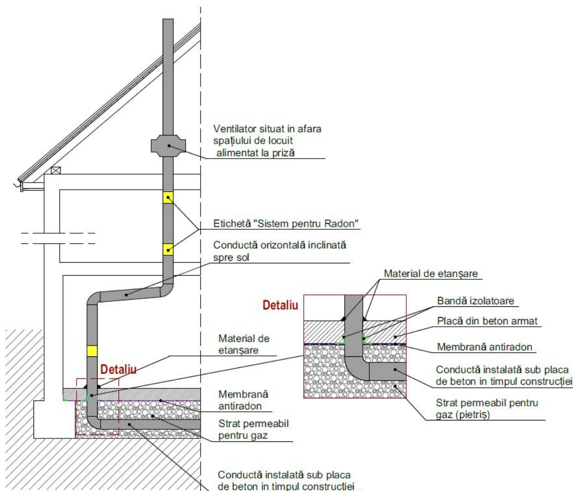
Figura 17 - Sistemul de depresurizare activă cu descărcare la nivelul acoperișului - Schema de principiu
