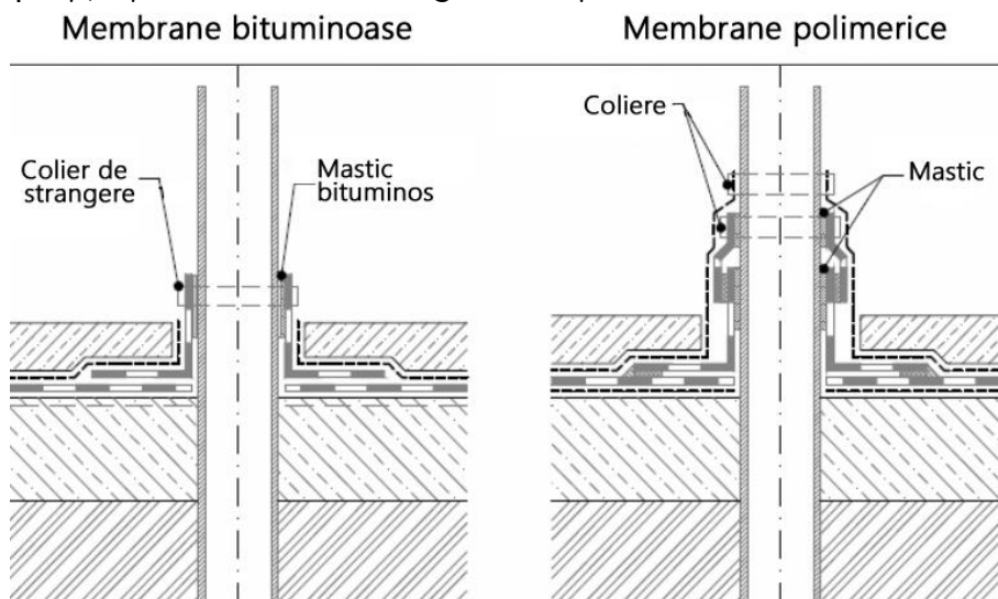
Figura 49 - Etanșarea golurilor de trecere pentru instalații.
