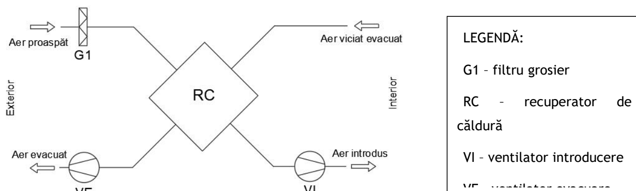
Figura 27 - Schemă de principiu și montaj sistem de ventilare mecanică descentralizată cu recuperare de căldură dublu-flux
