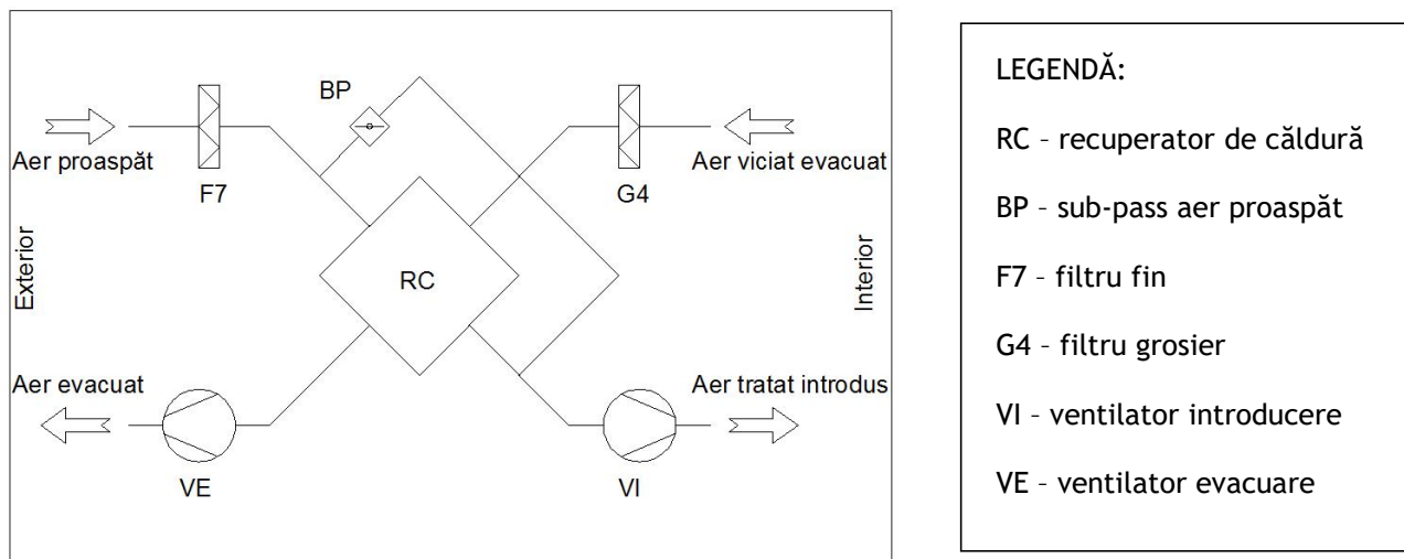
Figura 28 - Schema de principiu și montaj a echipamentului de ventilare mecanică centralizată cu recuperare de căldură (montaj în pod)
