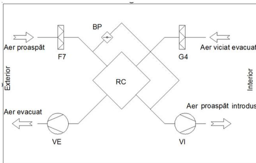
Figura 30 - Schemă de principiu echipament de ventilare mecanică centralizată cu recuperare de căldură (montaj pe perete)
