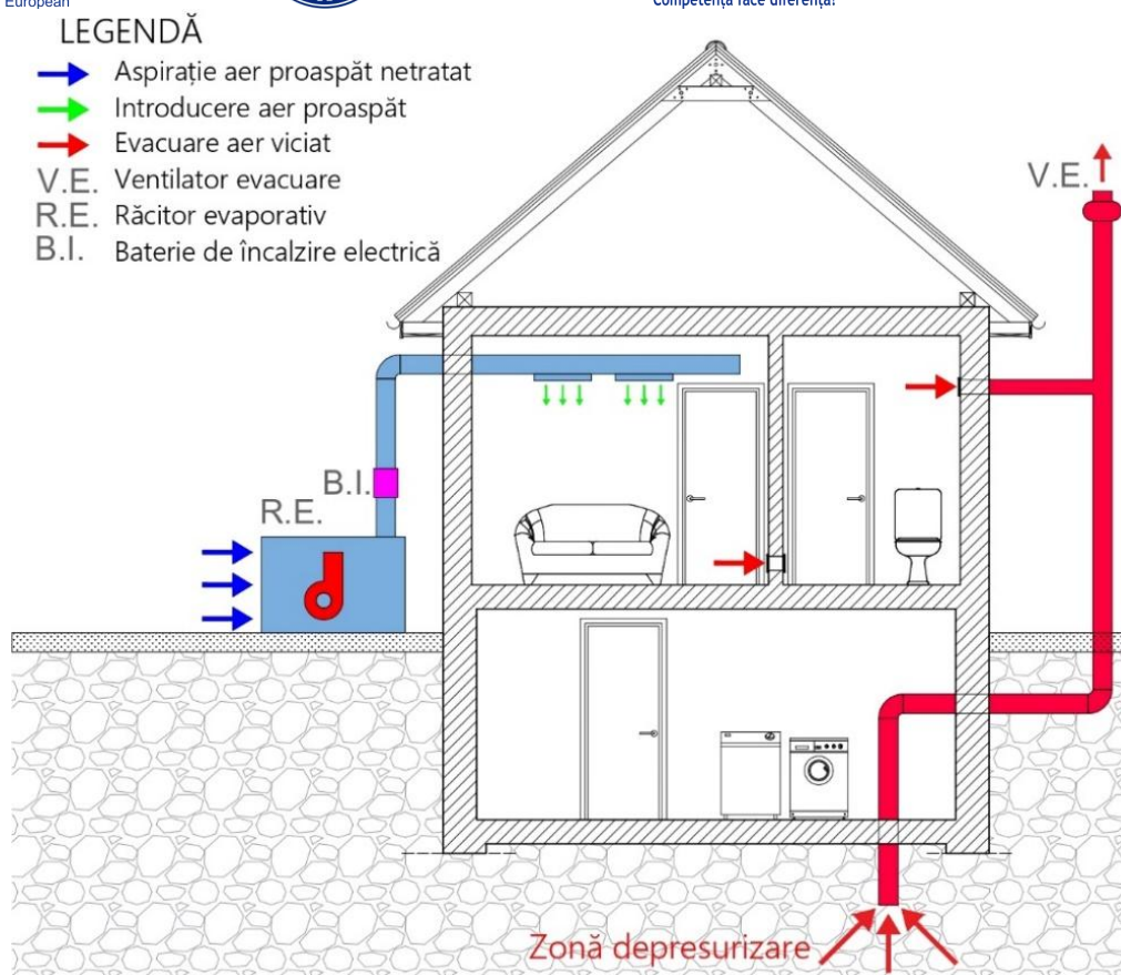
Figura 38 - Sistem de ventilație mecanică centralizată cu recuperare de căldură, depresurizare sol și răcitor evaporativ - Schema de principiu
