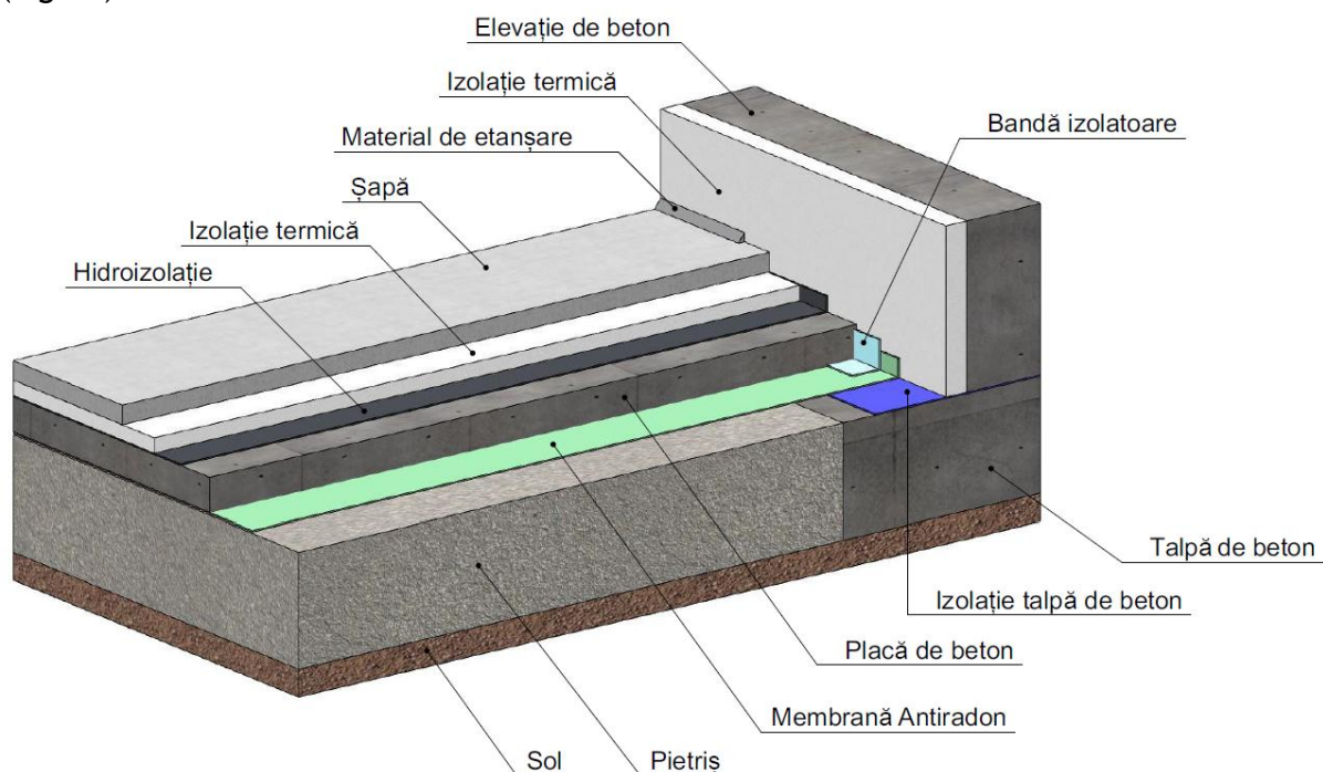
Fig. 5. Sigilarea de peretele fundației a membranei împotriva gazelor din sol - schema de principiu
