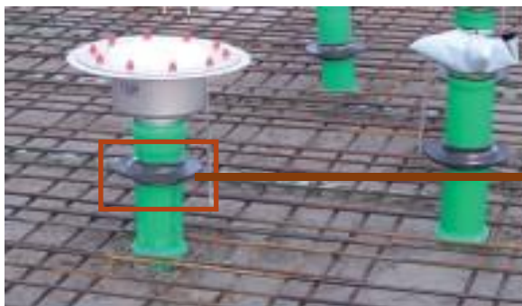
a. trecerea unei conducte de scurgere printr-o placă de fundație
