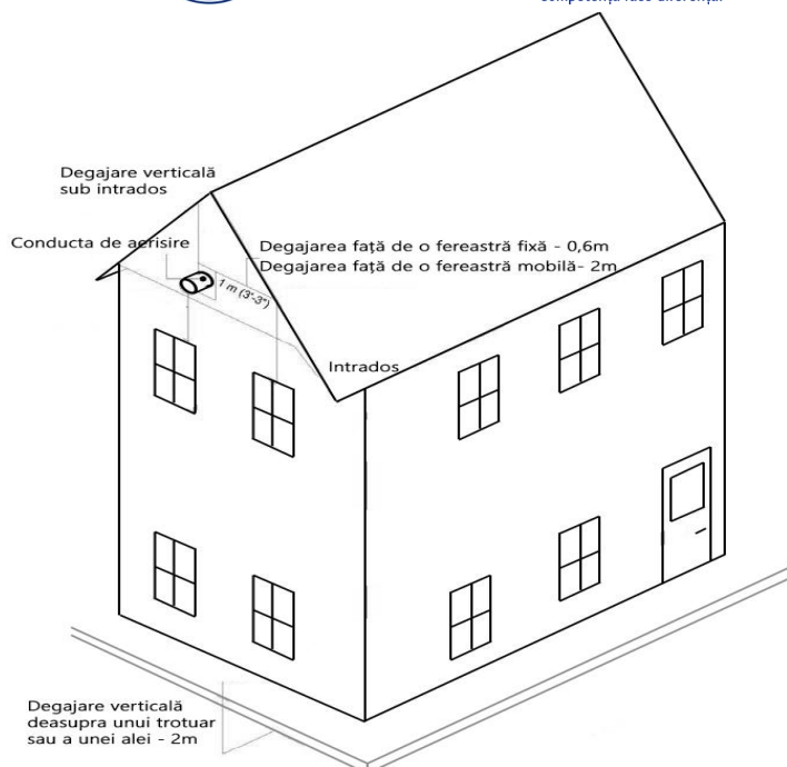
Fig. 8. Sistem de depresurizare activă cu descărcare la nivelul frontonului - schema de principiu
