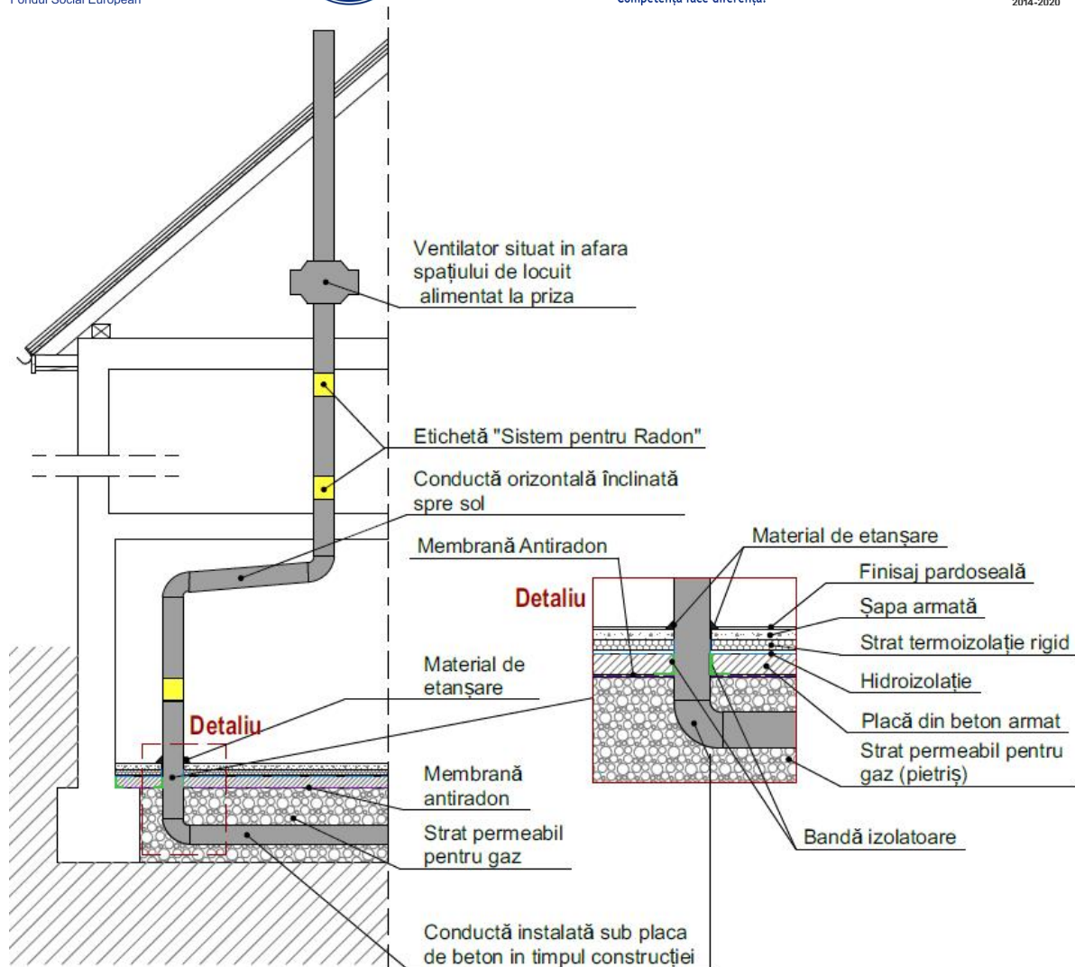
Fig. 7. Sistemul de depresurizare activă cu descărcare la nivelul acoperișului - schema de principiu
