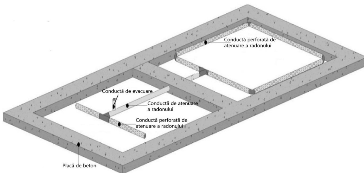
Fig. 4. Posibilă legătură a două straturi permeabile la gaze - schema de principiu
