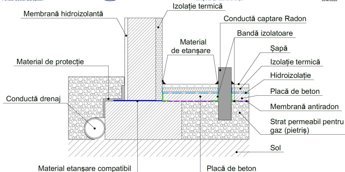
Fig. 6. Sigilarea orizontală a membranei împotriva gazelor din sol când izolația este între perete și placă - Schema de principiu
