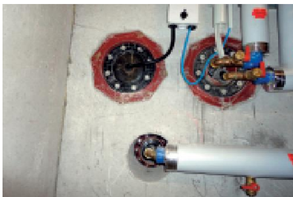
b. sistem etanș de conducte
