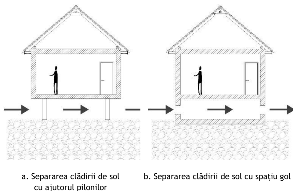
Fig. 1. Tipul clădirilor din perspectiva separării de terenul de fundare - schema de principiu
